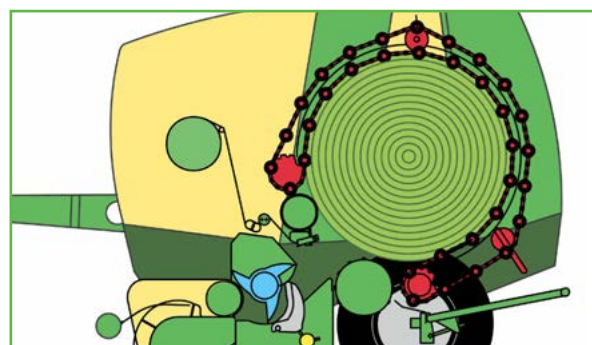
Variabele perskamer (V 1500 en V 1800): De twee eindloze kettingen met dwarsstaven vormen knalharde balen met hoge persdichtheid.
