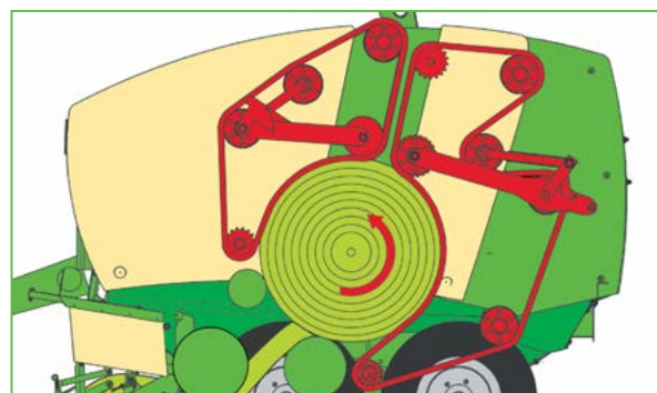
Variabele perskamer (V 1500 en V 1800): De twee eindloze kettingen met dwarsstaven vormen knalharde balen met hoge persdichtheid.
