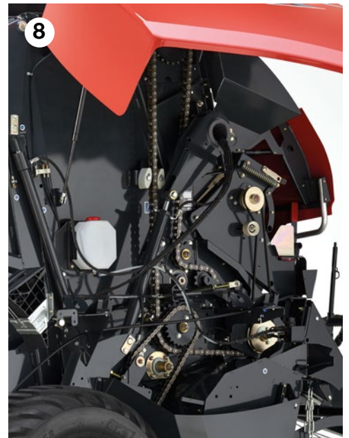
Robuust aandrijfsysteem met "IWIS"-kettingen van hoge kwaliteit + 1/4" 20BH hoofdaandrijving met hardverchroomde pennen
