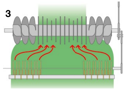
3 INTEGRAL ROTOR-technologie
